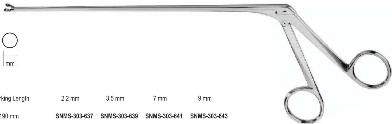
Oldberg SNMS-303-637 - SNMS-303-644
